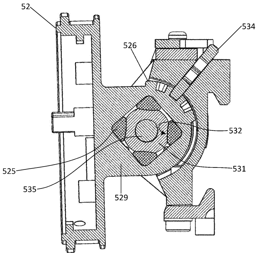
Section D-D
