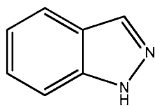
1H-indazole
