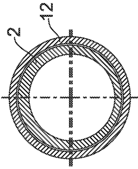
Section 'L-L' (1:6)
