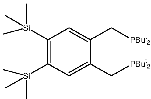
1,2-bis(di-tert-butyl(phosphinomethyl))-4,5- 5 bis(trimethylsilyl)benzene
