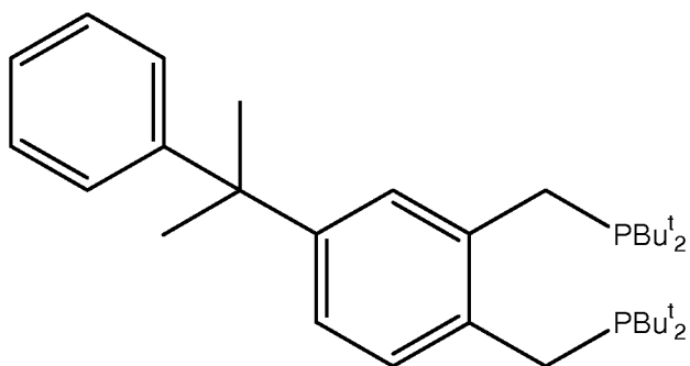
1,2-bis(di-tert-butyl(phosphinomethyl))-4-(2'-phenylprop-2'-yl)benzene
