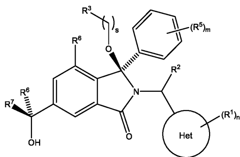
Diastereoisomer 2A
