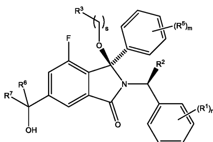
Diastereoisomer 1A
