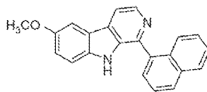
SP-141
