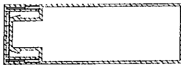
SECTION J-J FIG. 10B
