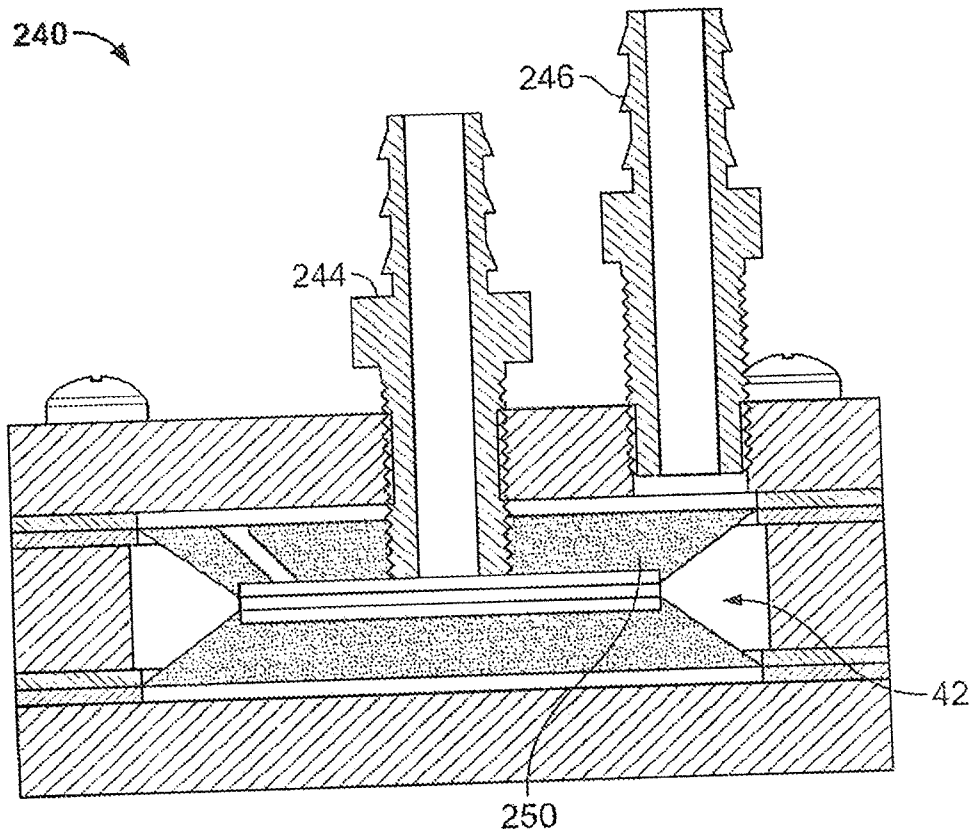
FIG. 24B
