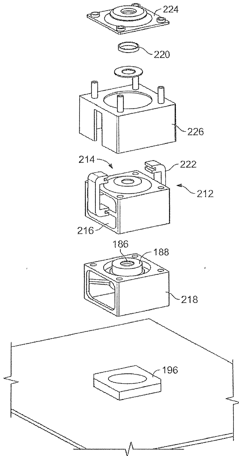
FIG. 21B
