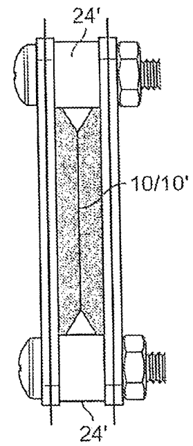
FIG. 9B
