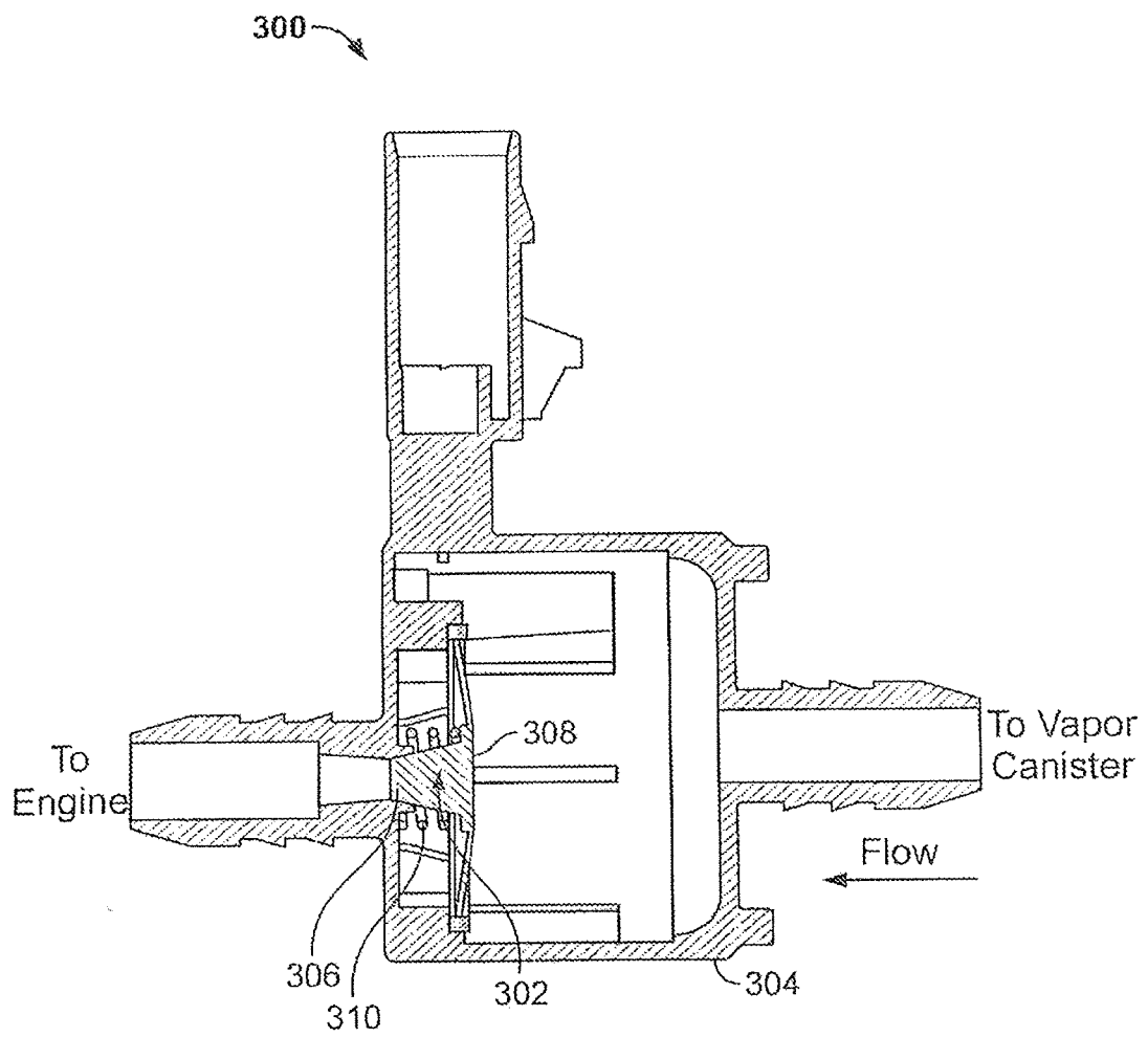
FIG. 30A
