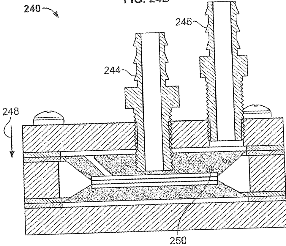
FIG. 24C
