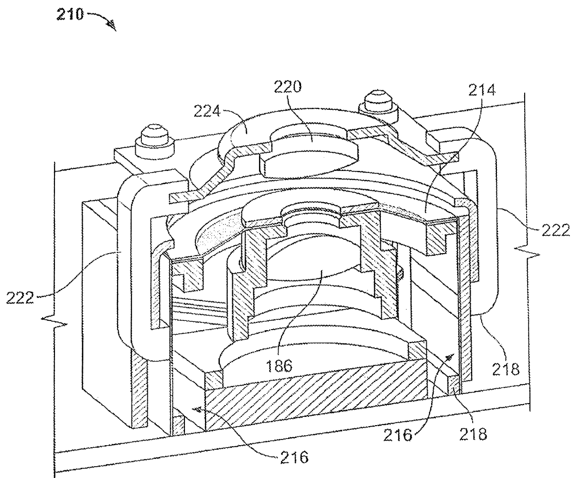
FIG. 21A
