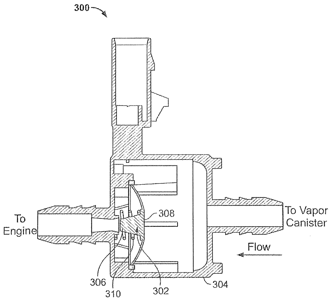
FIG. 30B
