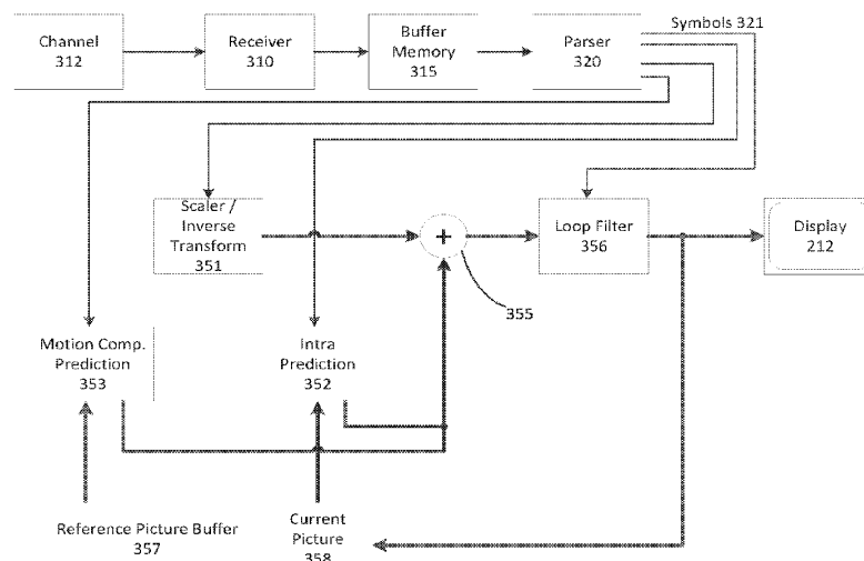
FIG. 3 Decoder 210
