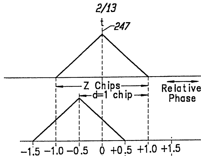
FIG. 5A (Punctual)
