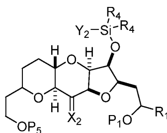
(VIII K),
