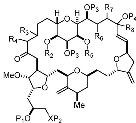
(IB),
