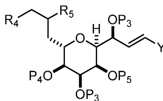
(IID),
