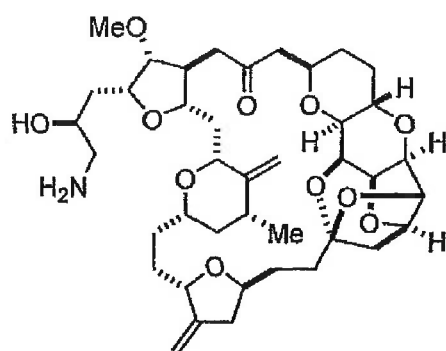
eribulin
