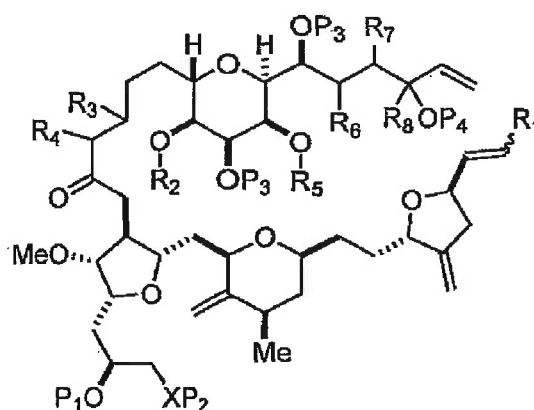
(IA),
