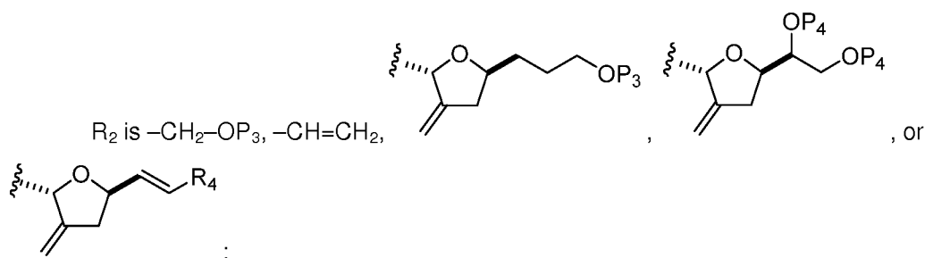
(VIIB),
