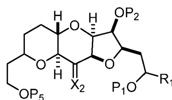
(VIIL),
