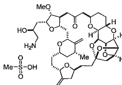
eribulin mesylate
