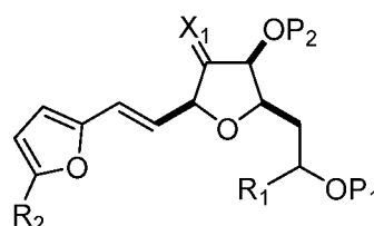
(VIII D);
