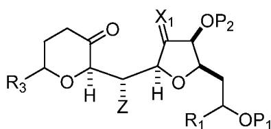
(VIII G);
