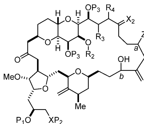
(IVB),
