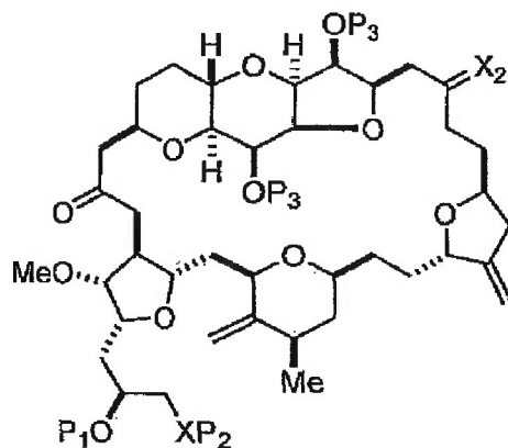
(ID);
