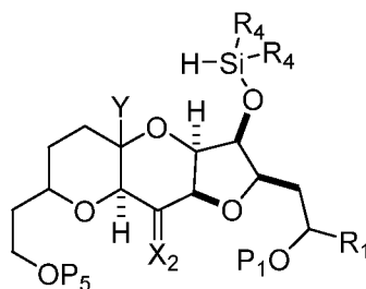
(VIII J),
