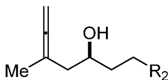
(VIIB),
