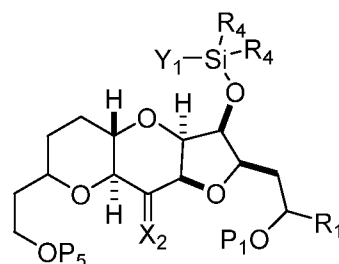
(VIIIK);
