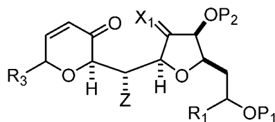
(VIII F),
