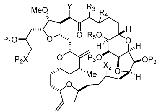
(VB),
