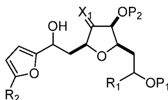
(VIII C) ,
