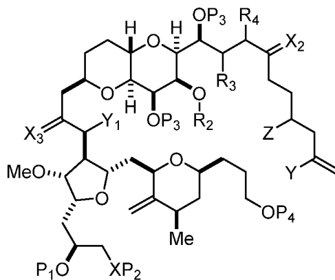
(IVD),
