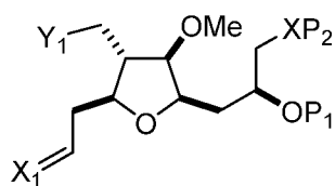
(VIIA),
