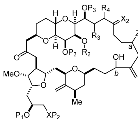
(IVB),
