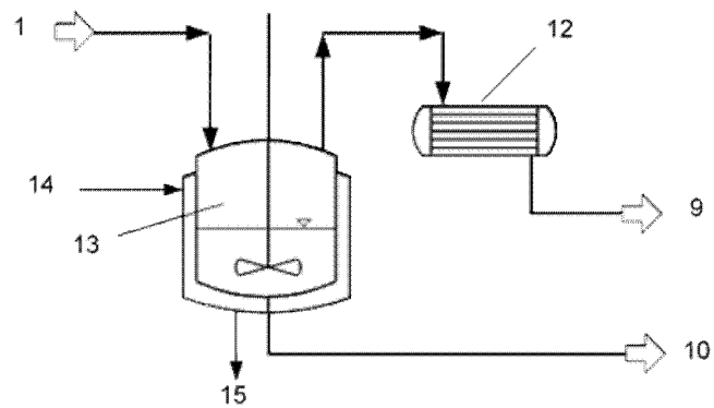
Figur 3: Diskontinuierliches Verfahren zur Gewinnung von 2-EHA.
