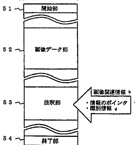
画像ファイルのフォーマット
