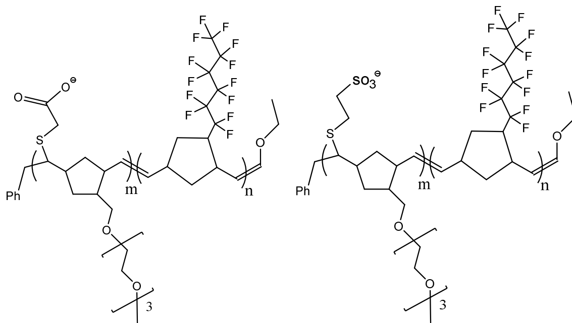
Poly(NTEG-b-NPF6)/MAcOH
