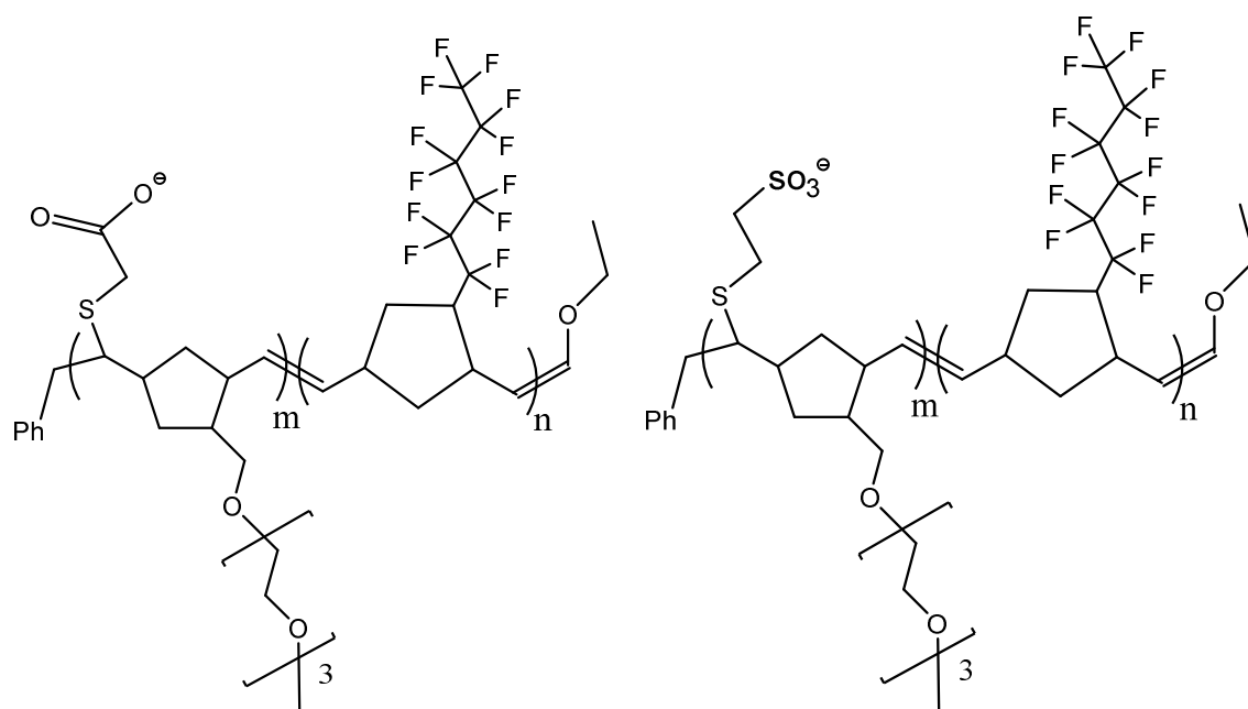
Poly(NTEG-b-NPF6)/MAcOH
