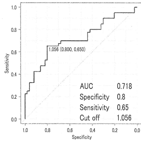
SerpinA3-SerpinA3
