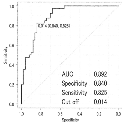
SerpinA3-SerpinA3
