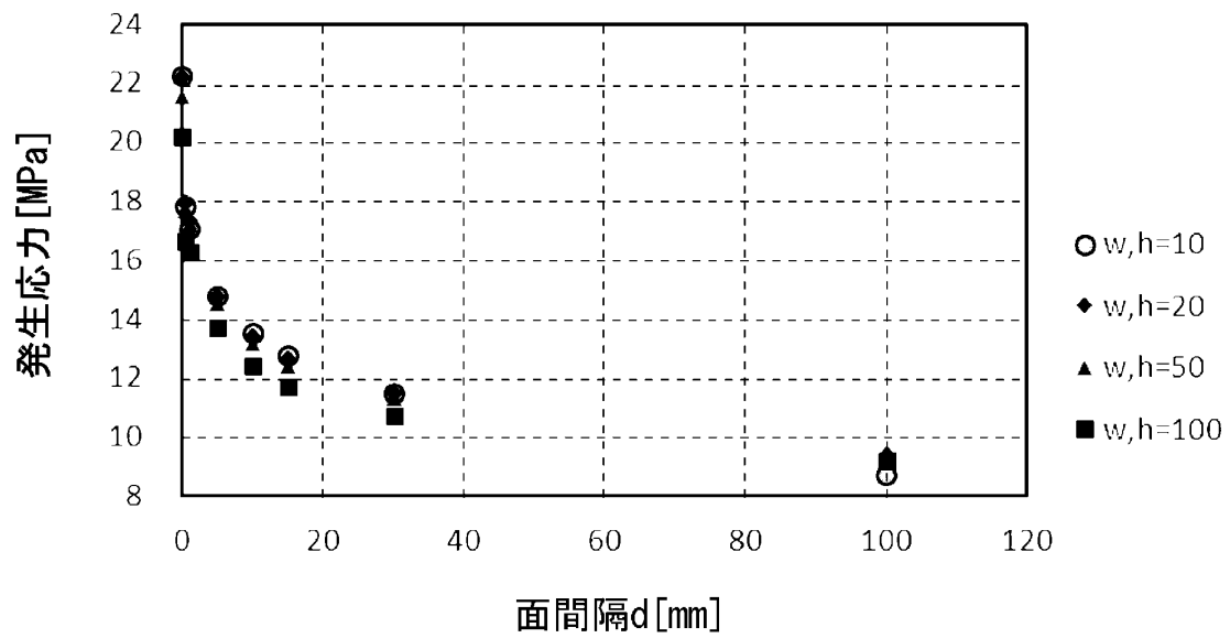
面間隔dと発生応力の関係
