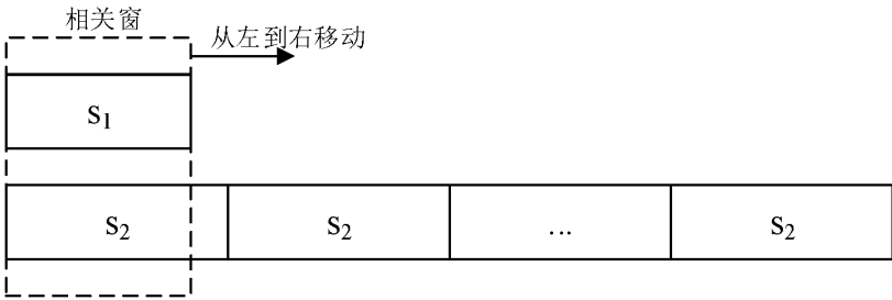
(b) s_1 和 s_2 不相同，CIR计算示意图
