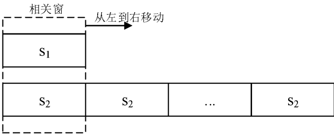
(a) s_1 和 s_2 相同时，CIR计算示意图
