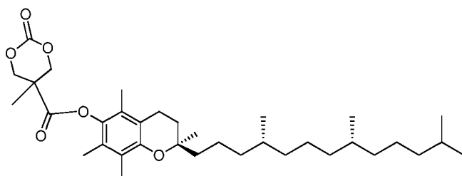
MTC-VitE
