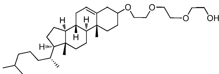
(Chol-OPrOH),
