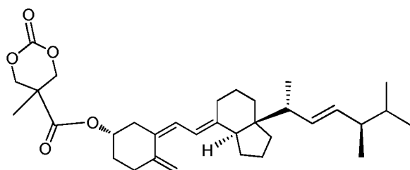
MTC-VitD2
