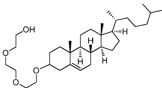
Chol-OTEG-OH
