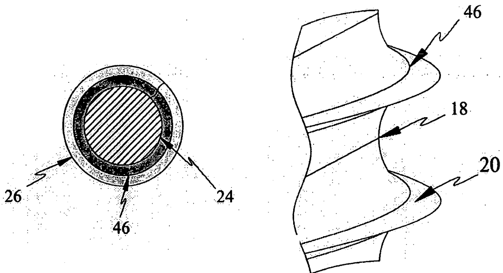
SECTION A-A FIG. 1B
