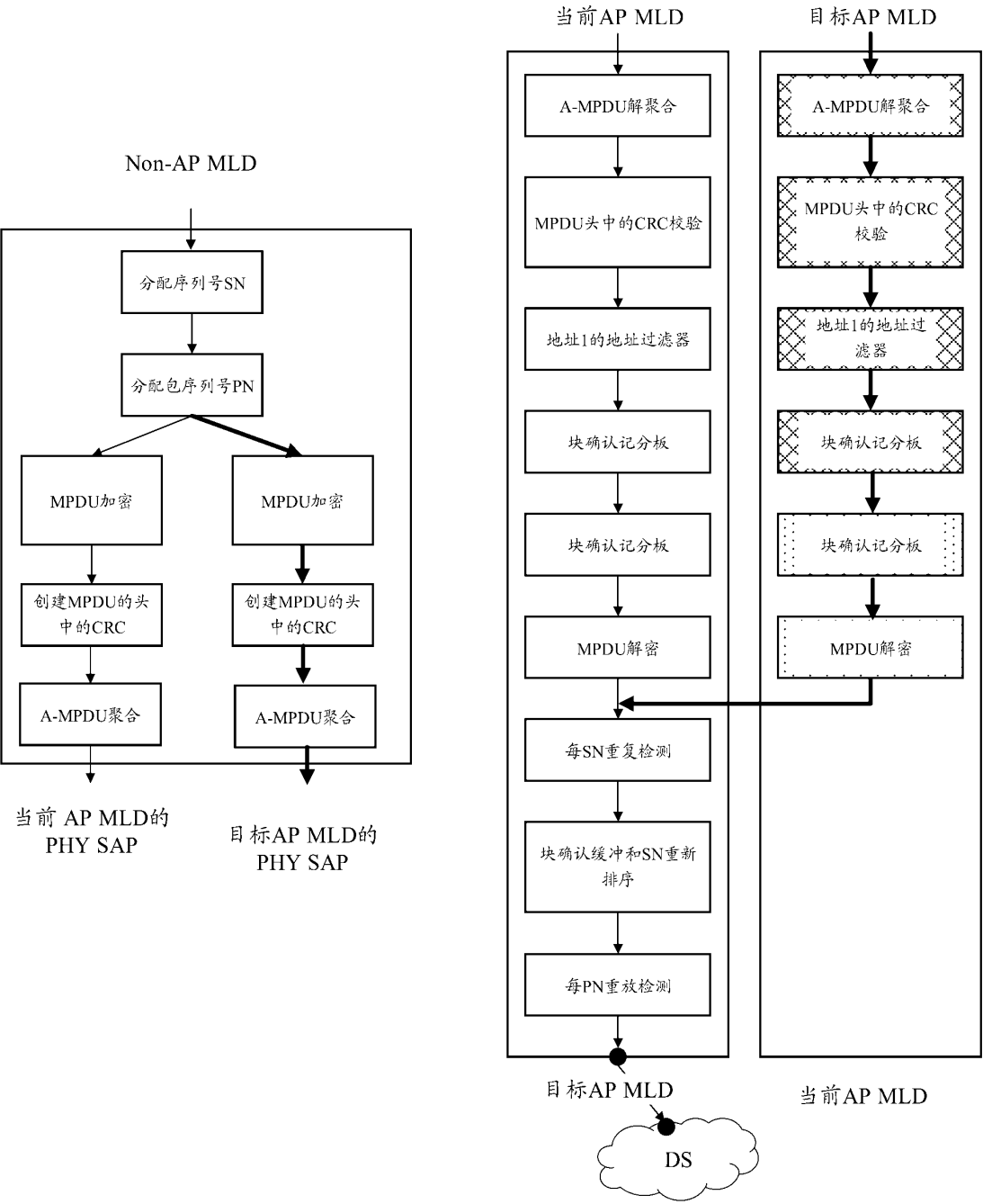
上行发送端处理流程示意图
