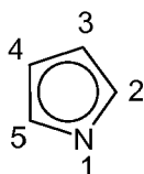
azacyclopentadienyl
