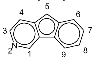
indeno[1,2-c]pyridyl
