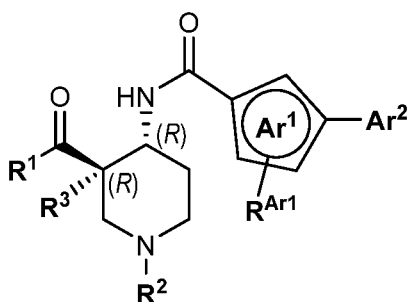
Formula (I R )
