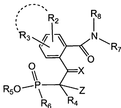
Formula (D)
