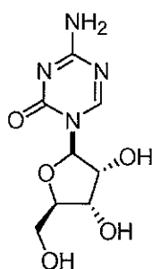
5-azacytidine
