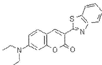
Coumarin 6
