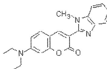
Coumarin 30
