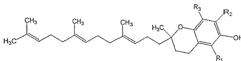
Tocotrienol
