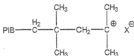
PIB Carbenium Ion
