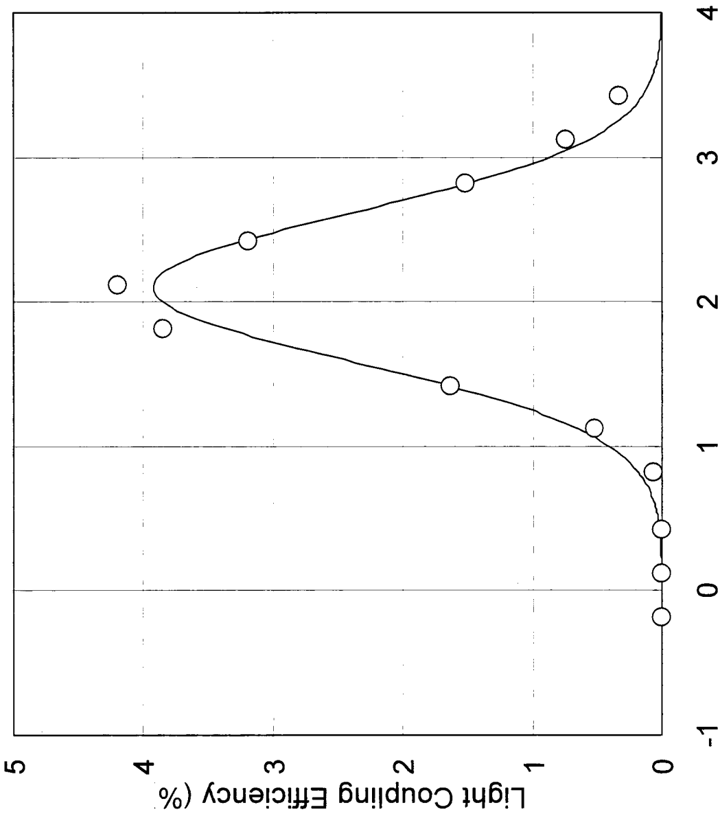
Fig. 6 Log 10 (MFP)
