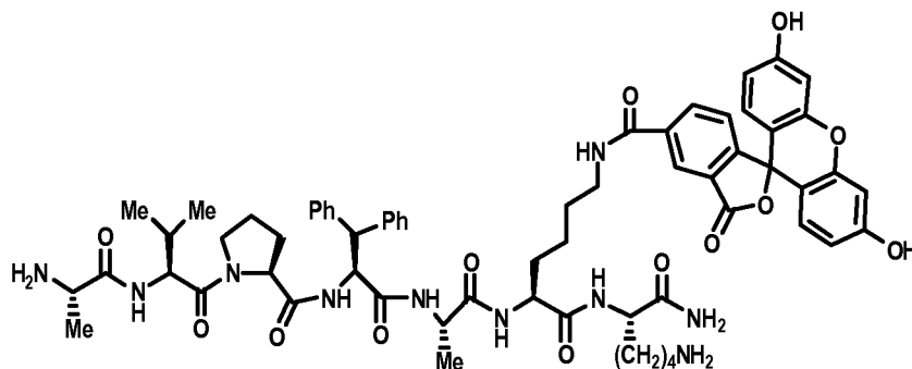
AVP-diPhe-FAM probe
