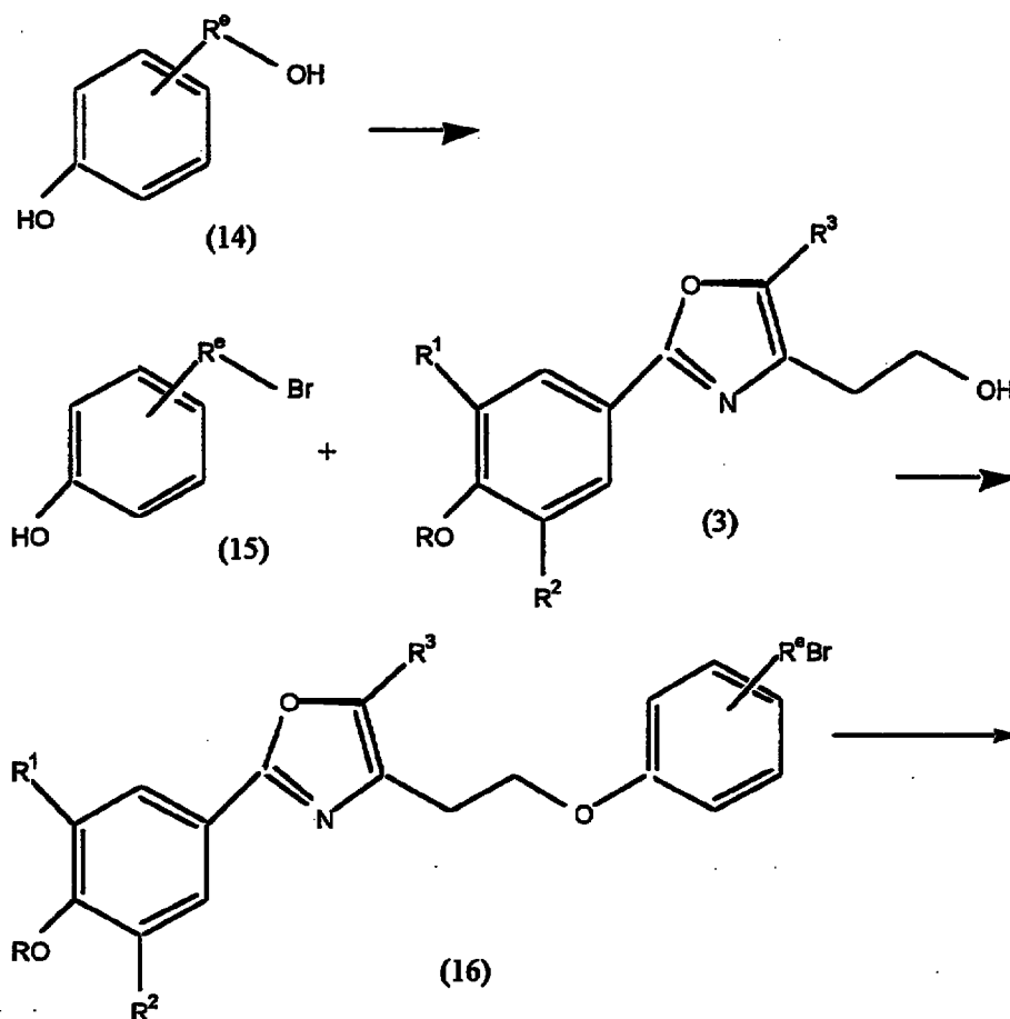
Scheme I(d)
