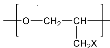
(1P)
