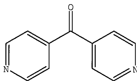
4,4'-dipyridylketone
