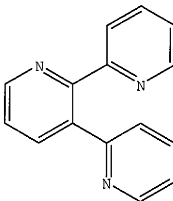
terpyridine
