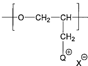
(1N)
