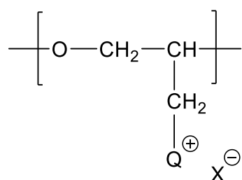
(1N)
