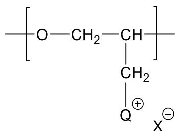
(1N)
