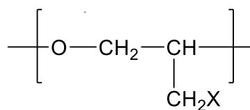
(1P)
