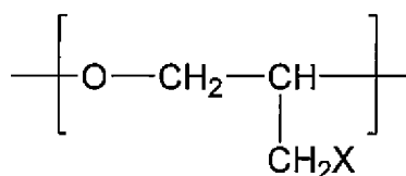
(1P)
