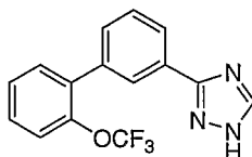
3-[3-(2-Trifluoromethoxyphenyl)-phenyl]-1,2,4-triazole
