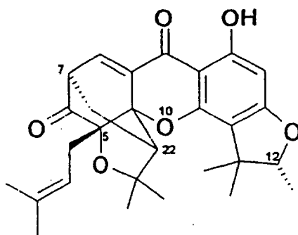
Sootepenseone
