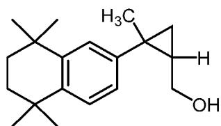
(XIa),
