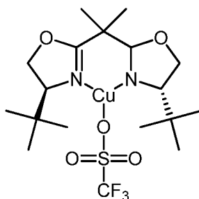
(XIX)
