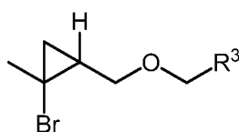
(VIIIa),
