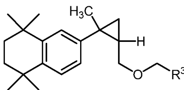
(Xa),
