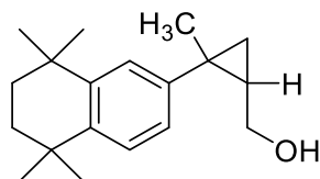
(XIa),
