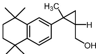
(XIa),
