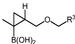
(IXa),
