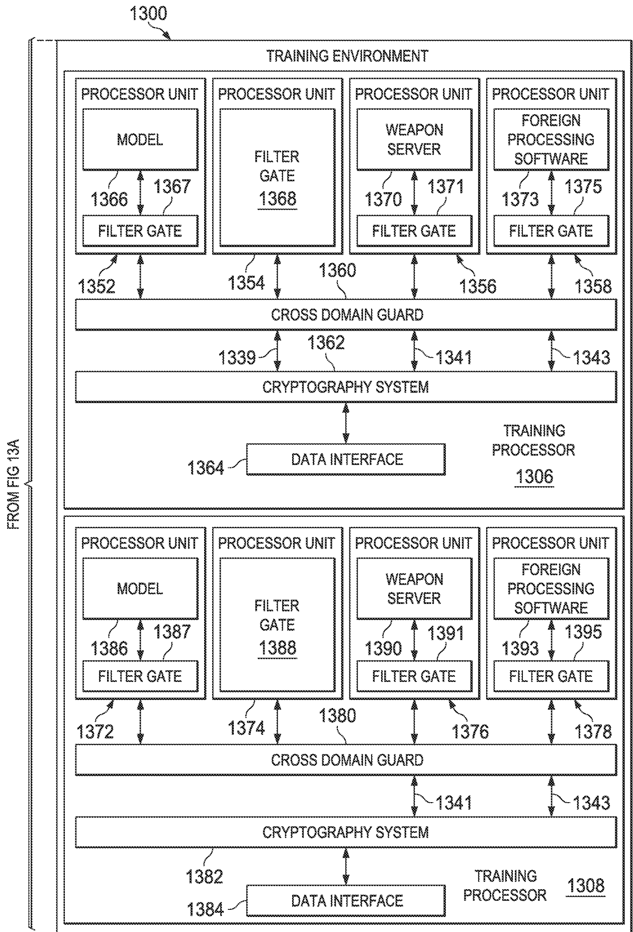
FIG. 13B
