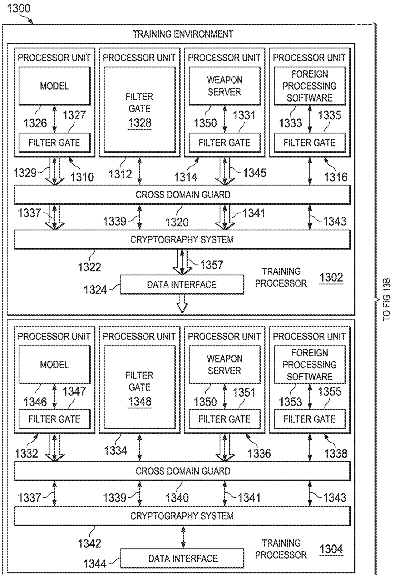
FIG. 13A
