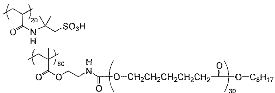
(B-1-5) Mw 42,000
