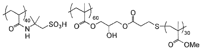
(B-1-7) Mw 36,000
