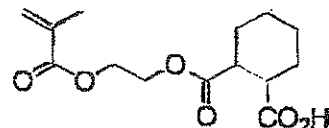
Monomer e
