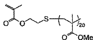
Macromonomer (1-3)
