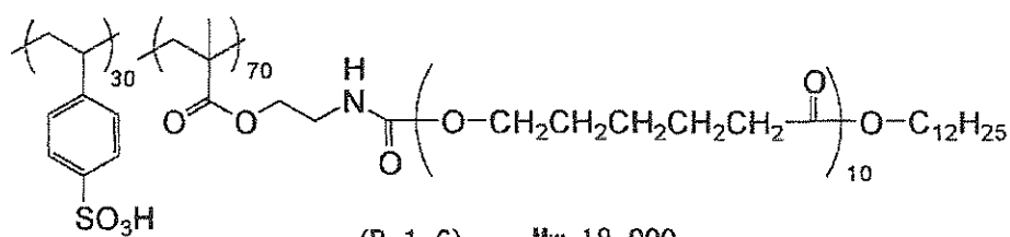
(B-1-6) Mw 18,000
