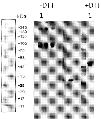
1 MX1 IL-17A-mFc
