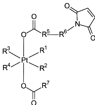
(Ij)
