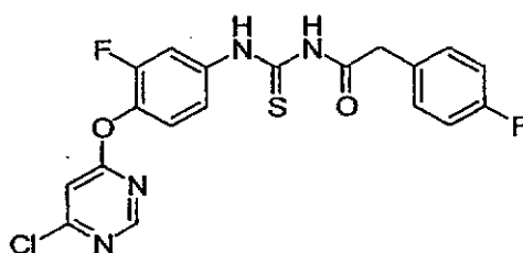
1-(4-(6-Chloropyrimidin-4-yloxy)-3-fluorophenyl)-3-(2-(4-fluorophenyl)acetyl) thiourea
