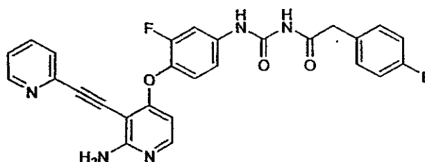
1-(4-(2-Amino-3-(2-(pyridin-2-yl)ethynyl)pyridin-4-yloxy)-3-fluorophenyl)-3-(2-(4-fluorophenyl)acetyl)urea, dihydrochloride salt
