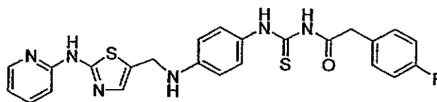
1-(2-(4-Fluorophenyl)acetyl)-3-(4-((2-(pyridin-2-ylamino)thiazol-5-yl)methylamino)phenyl)thiourea
