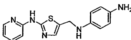
1-(2-(4-Fluorophenyl)acetyl)-3-(4-((2-(pyridin-2-ylamino)thiazol-5-yl)methylamino)phenyl)thiourea
