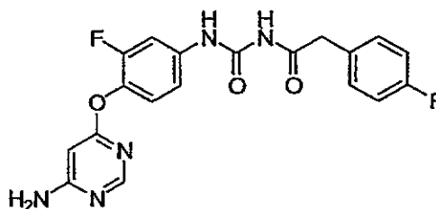
1-(4-(6-Aminopyrimidin-4-yloxy)-3-fluorophenyl)-3-(2-(4-fluorophenyl)acetyl)urea
