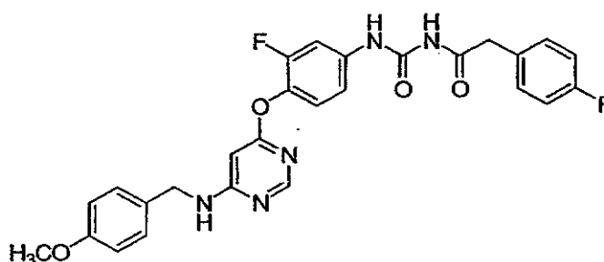
1-(4-(6-(4-Methoxybenzylamino)pyrimidin-4-yloxy)-3-fluorophenyl)-3-(2-(4-fluorophenyl)acetyl)urea
