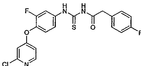
1-(4-(2-Chloropyridin-4-yloxy)-3-fluorophenyl)-3-(2-(4-fluorophenyl)acetyl)thiourea
