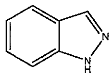
1H-indazole
