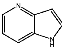
1H-pyrrolo[3,2- b ]pyridine
