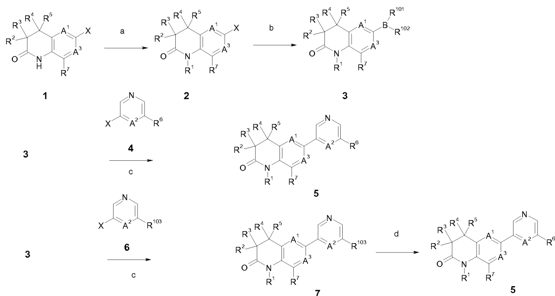
Scheme 1a
