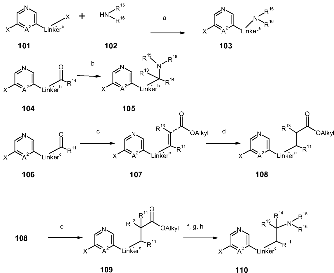
Scheme 2a
