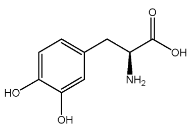
L-DOPA
