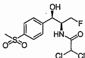
Florfenicol
