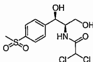
Thiamphenicol
