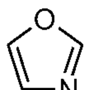
oxazole (oxazolyl)
