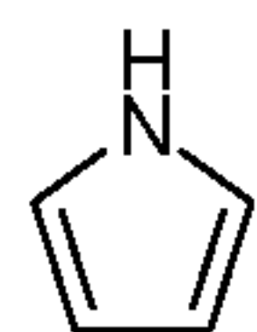
pyrrole (pyrrolyl)
