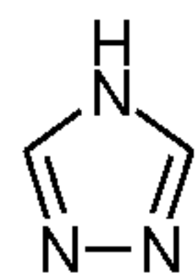
1,3,4-triazole (1,3,4-triazolyl)
