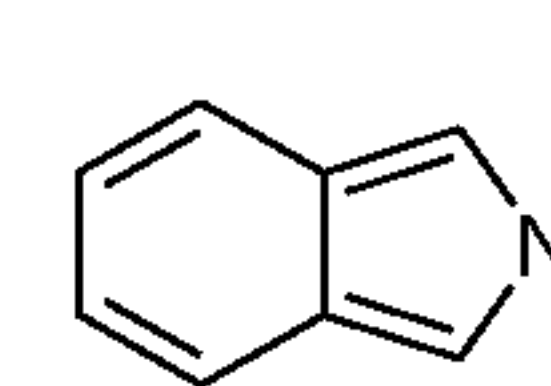
isoindole (isoindolyl)
