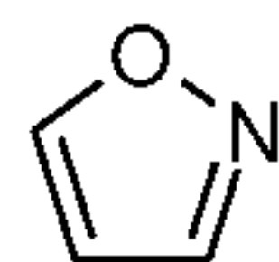
isoxazole (isoxazolyl)
