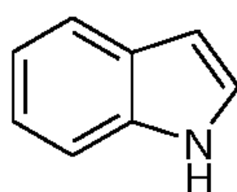
indole (indolyl)
