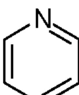
pyridine (pyridinyl)
