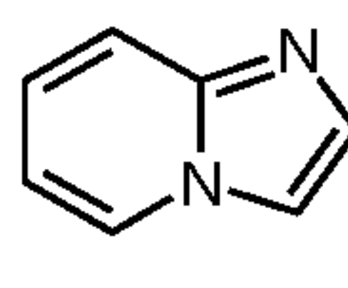
imidazo[1,2-a]pyridine (imidazo[1,2-a]pyridinyl)
