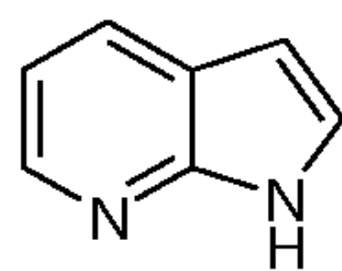
pyrrolo[2,3-b]pyridine (pyrrolo[2,3-b]pyridinyl)
