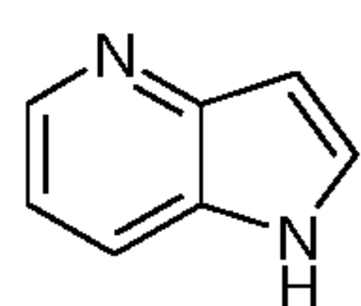
pyrrolo[3,2-b]pyridine (pyrrolo[3,2-b]pyridinyl)
