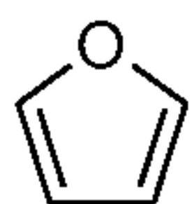
furan (furanyl)
