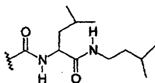
[-CO-leucyl-NH-isoamyl]
