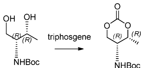
N-Boc-L-threoninol L-tBuMODC
