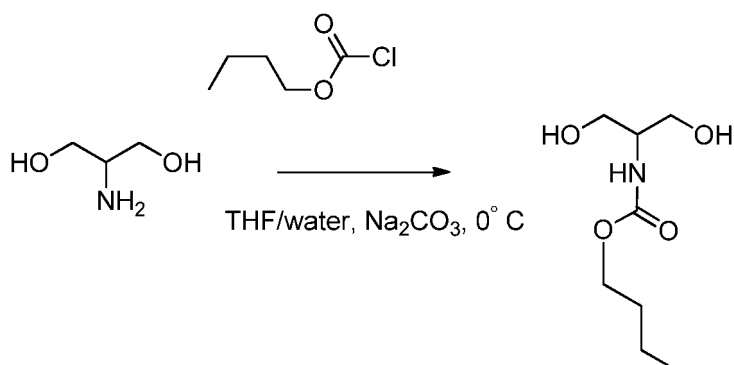
Serinol
