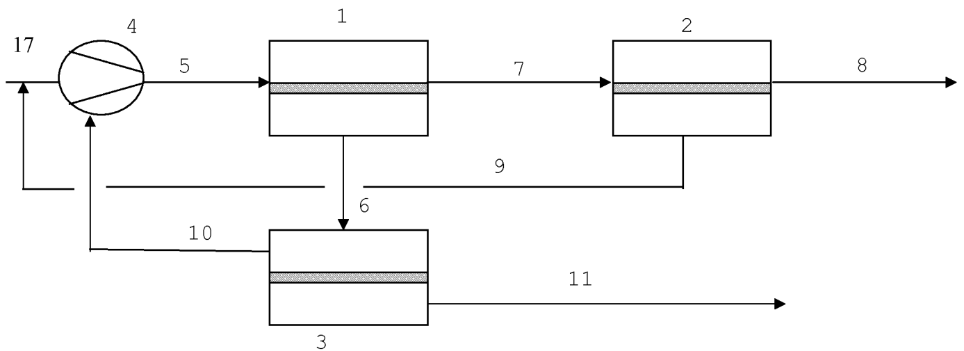
Abb. 2: 3-Stufige Verschaltung von Membranmodulen mit 10 einem Kompressor und Retentatrückführung der Membrantrennstufe (3) ohne Drosselung in eine erhöhte Kompressionsstufe
