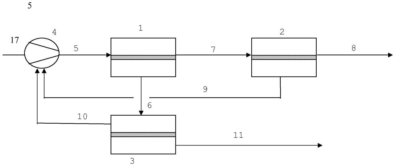
10 Abb. 3: 3-Stufige Verschaltung von Membranmodulen mit einem Kompressor und Retentatrückführung der dritten Stufe ohne Drosselung sowie Permeatrückführung der zweiten Stufe in eine erhöhte Kompressionsstufe
