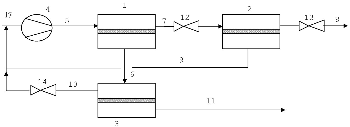
Abb. 1: Beispielhafte Verschaltung von mehreren 5 Membranmodulen laut Erfindung
