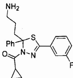
[2-(3-Aminopropyl)-5-(3-fluorophenyl)-2-phenyl-[1,3,4]thiadiazol-3-yl]- cyclopropylmethanone
