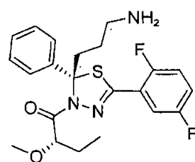
(Enantiomer A)
