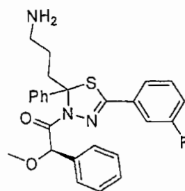
(Diastereomer A)
