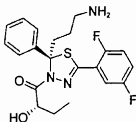
(S)-1-((R)-2-(3-aminopropyl)-5-(2,5-difluorophenyl)-2-phenyl-1,3,4-thiadiazol-3(2H)-yl)-2-hydroxybutan-1-one
