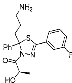
(Diastereomer A)
