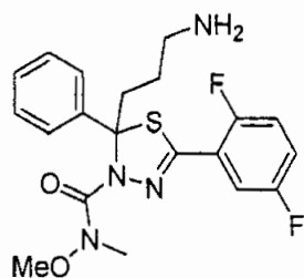
(Enantiomer A)
