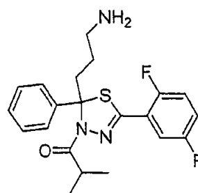
(Enantiomer A)
