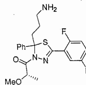
(Diastereomer A)
