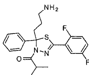
(Enantiomer B)
