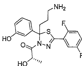
(Diastereomer A)
