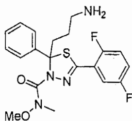
(Enantiomer B)
