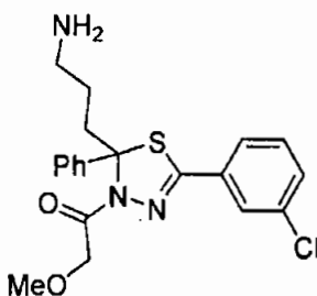
1-(2-(3-Aminopropyl)-5-(3-chlorophenyl)-2-phenyl-1,3,4-thiadiazol-3(2H)-yl)-2- methoxyethanone
