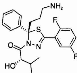
(S)-1-((S)-2-(3-aminopropyl)-5-(2,5-difluorophenyl)-2-phenyl-1,3,4-thiadiazol-3(2H)-yl)-2-hydroxy-3-methylbutan-1-one
