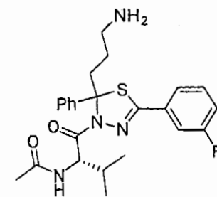
(Diastereomer A)
