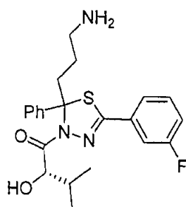
(Diastereomer A)
