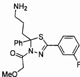
1-[2-(3-Aminopropyl)-5-(3-fluorophenyl)-2-phenyl-[1,3,4]thiadiazol-3-yl]-2- methoxyethanone
