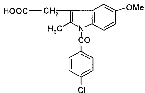
Indomethacin
