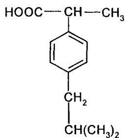
Ibuprofen
