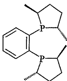
( S,S )-Me-DuPhos
