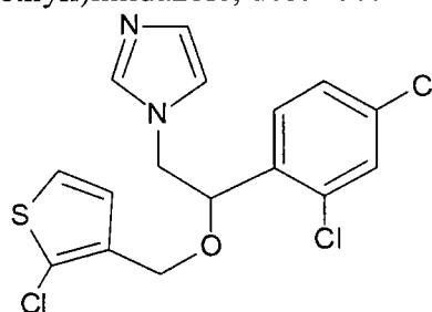
Tioconazole
