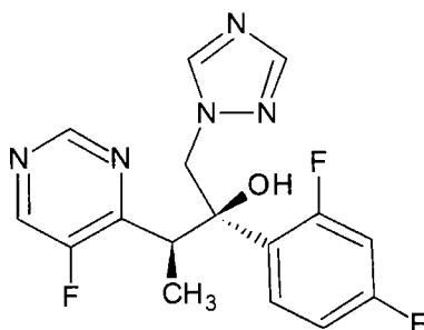
Voriconazole
