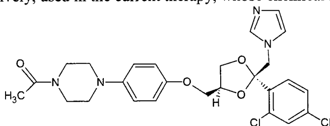
Ketoconazole
